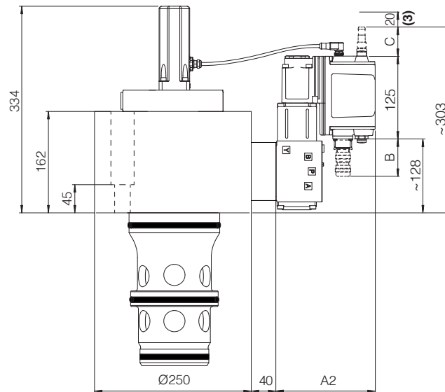
LIQZP-LEB-803 LIQZP-LES-803
