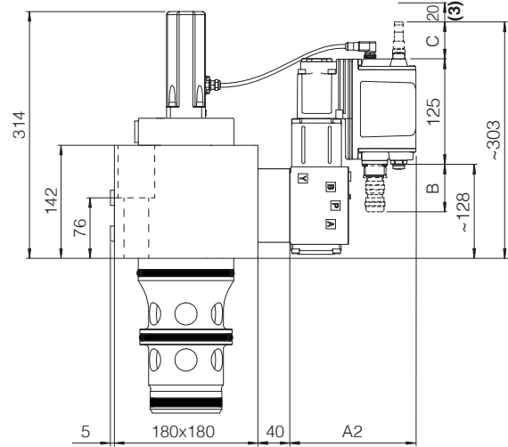
LIQZP-LEB-633 LIQZP-LES-633
